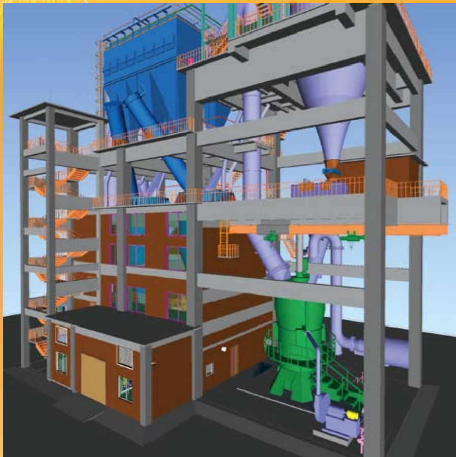
三维设计煤磨模型
